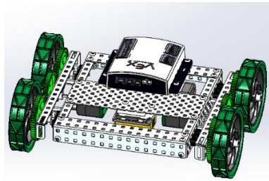
VEX 小车底盘零件的装配关系
